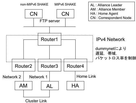
図 8 実験環境
